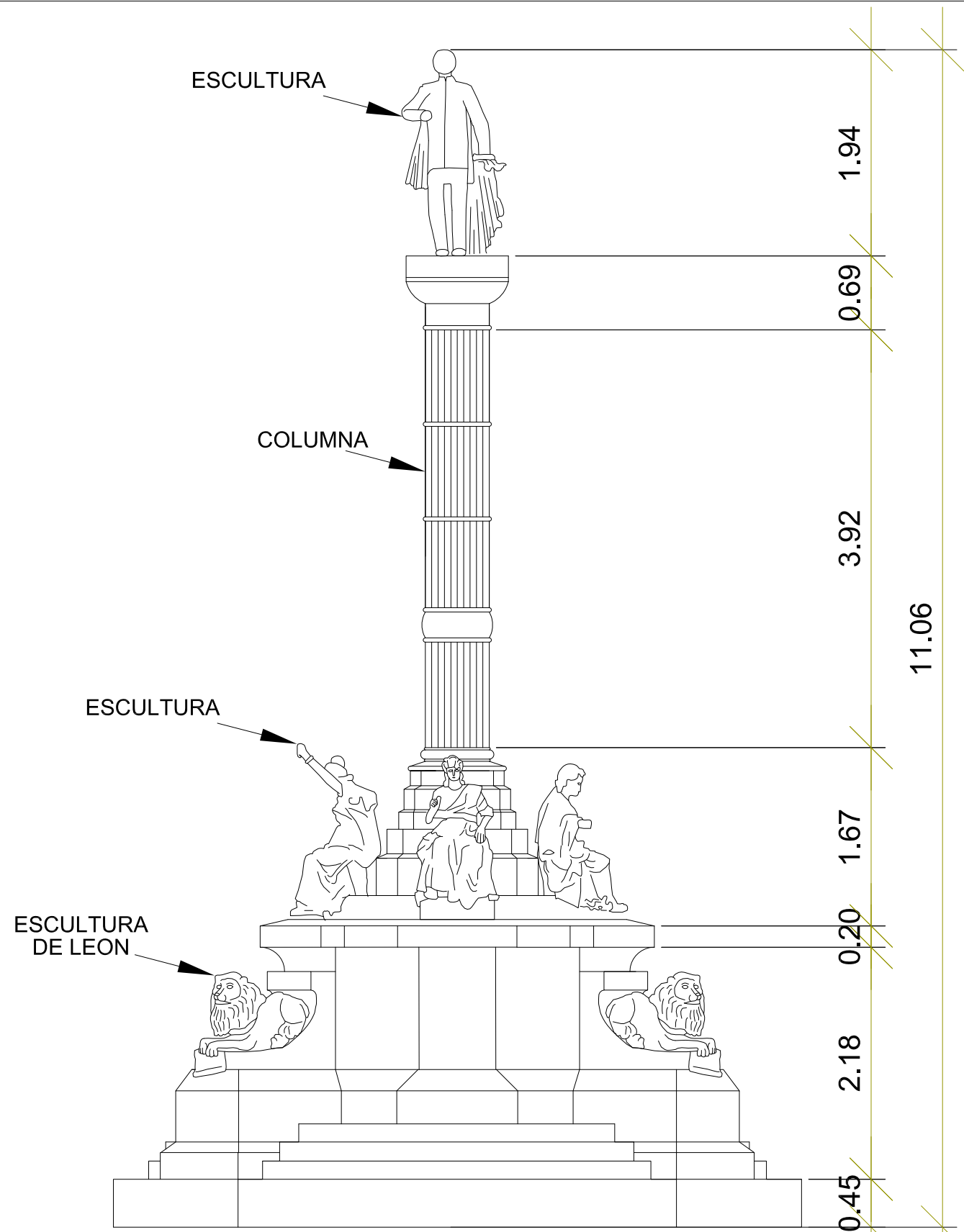
ELEVACION MONUMENTO A MIGUEL GARCIA GRANADOS ESCALA 1:50
