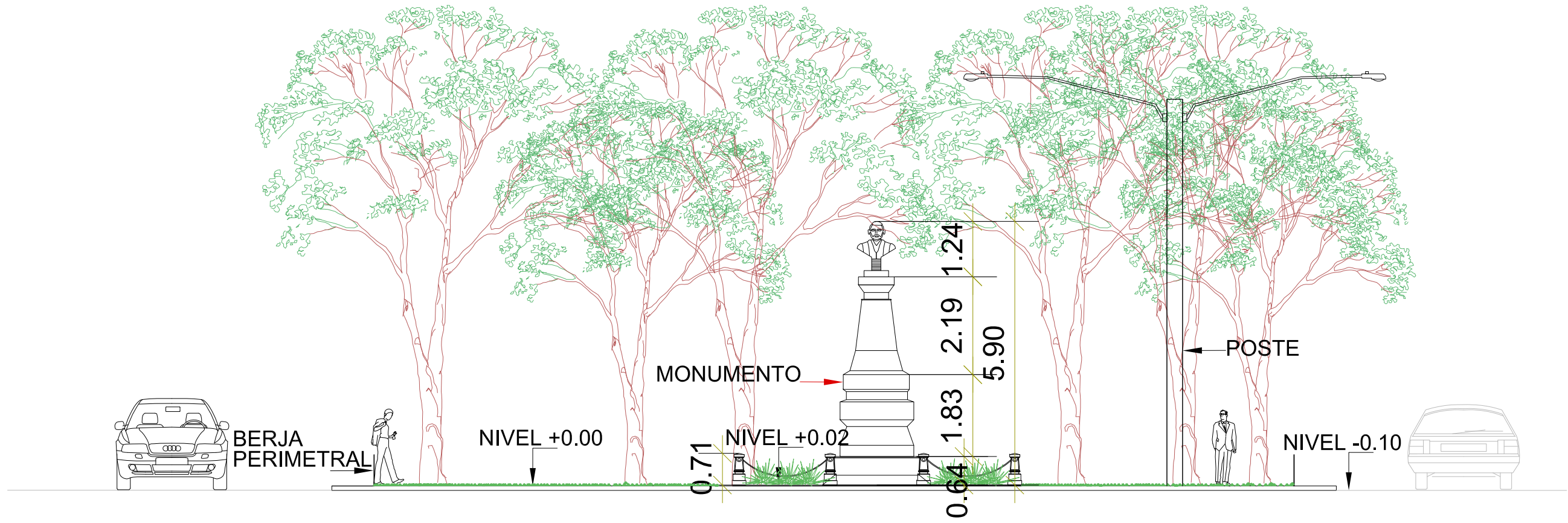
ELEVACION MONUMENTO A BENITO JUAREZ ESCALA 1:100
